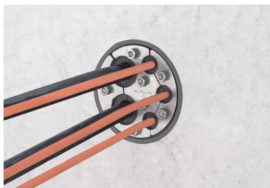
HRD 100 SG 2x8-30+3x4-16,5 v zabetonované pažnici
